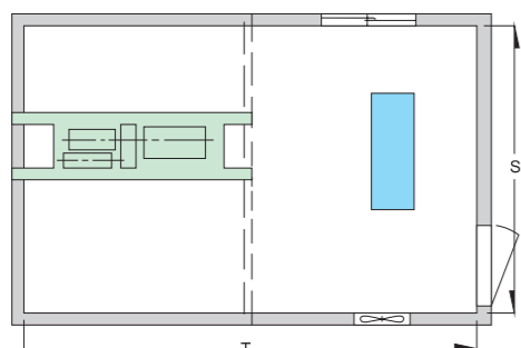
機械室平面圖
