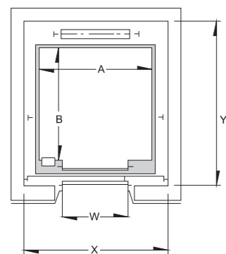
升降路平面圖
