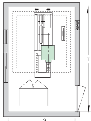
機械室平面圖
