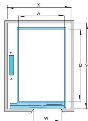
升降路平面圖
