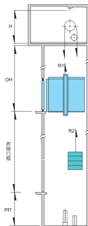
升降路斷面圖
