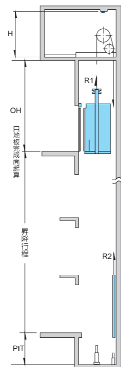
升降路斷面圖
